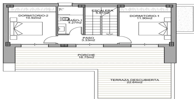
PLANTA PRIMERA
